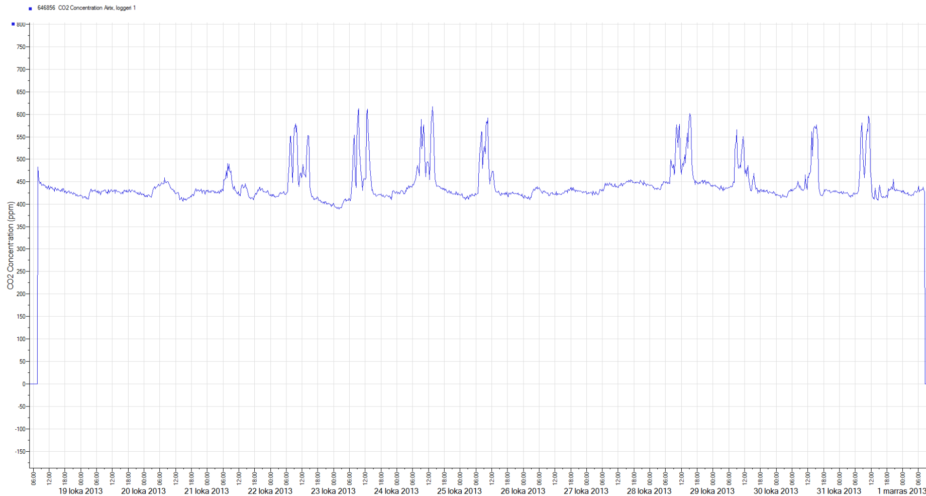
Kuva 1. Huoneen 207 CO2-pitoisuustulokset 16.10-31.10 ajalta.
