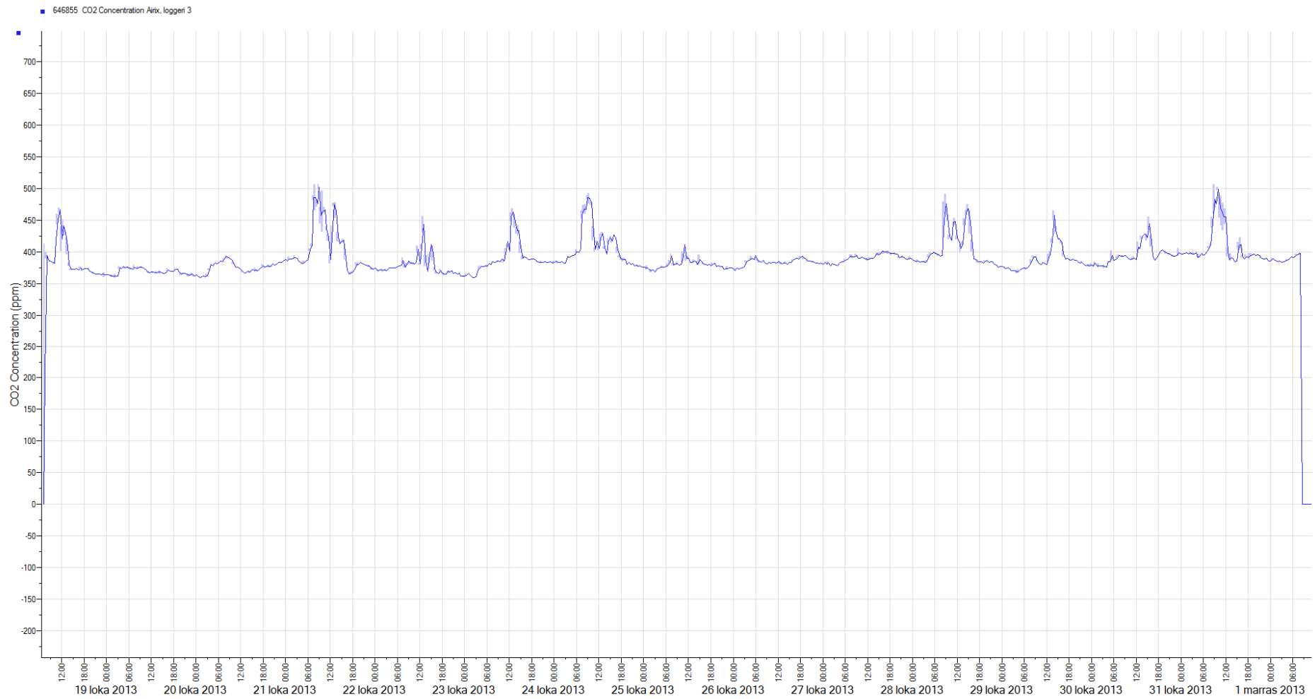
Kuva 4. Huoneen 261 CO 2 -pitoisuustulokset 16.10-31.10 ajalta.
