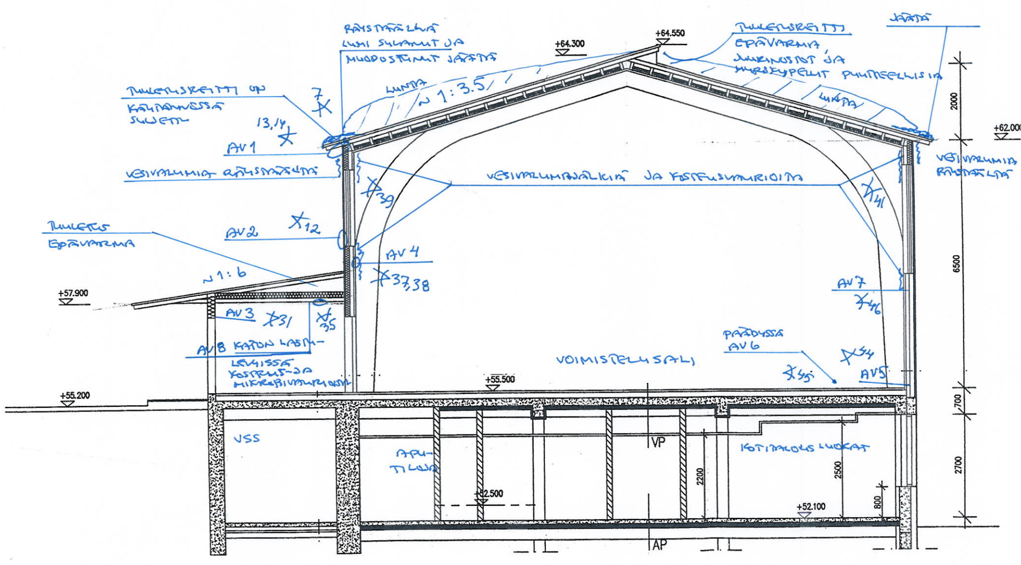
LEIKKAUS A-A
