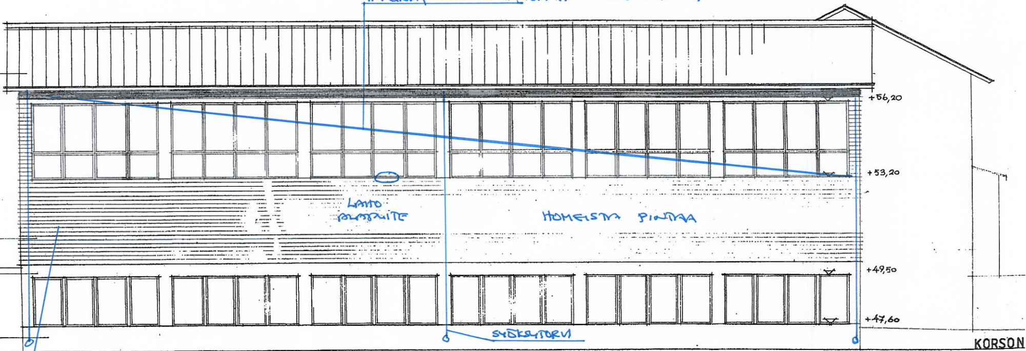
JULKISIVU POHJOISEEN
