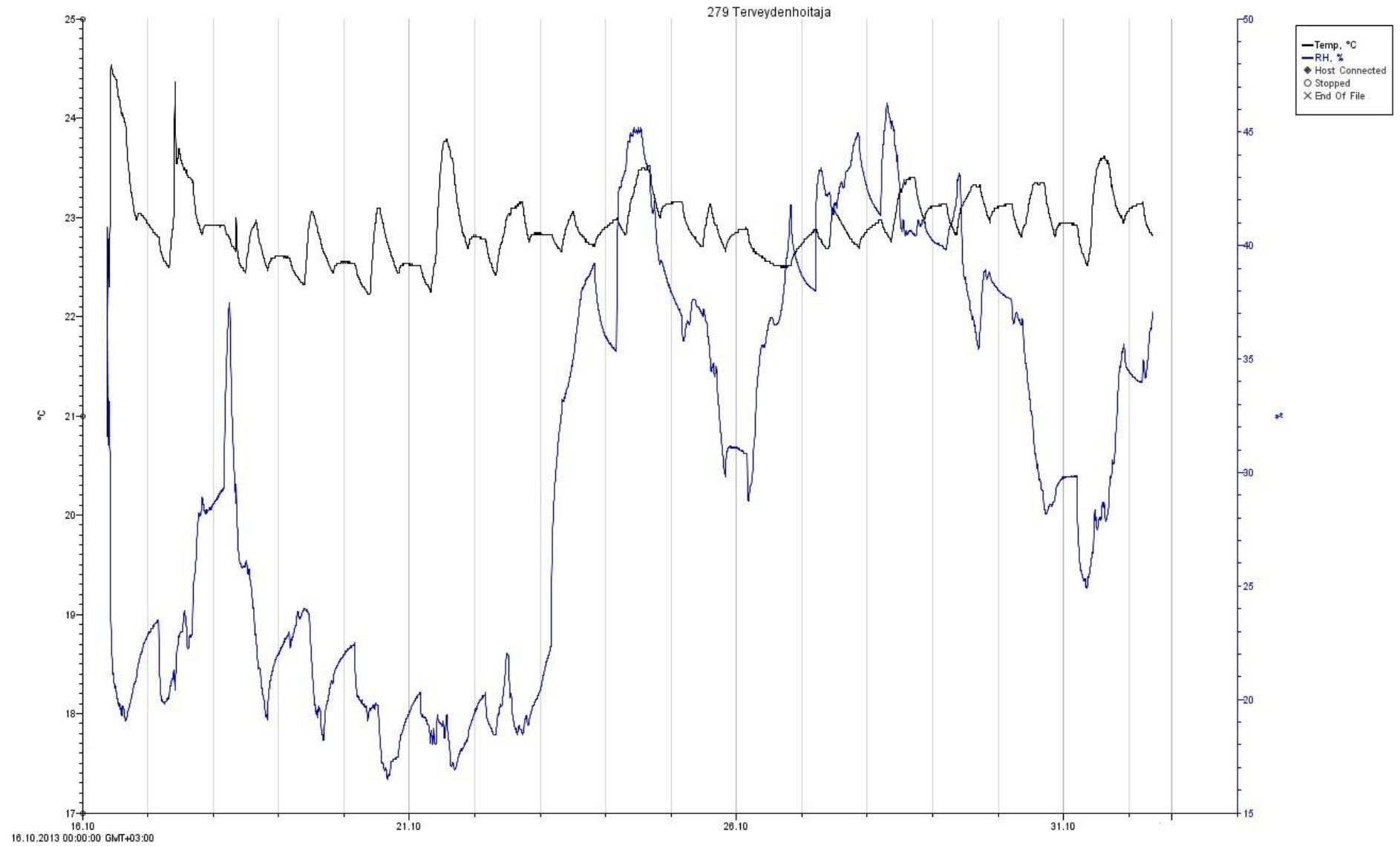
Kuva 8. Huoneen 279 Lämpötila- ja kosteustulokset 16.10-31.10 ajalta.
