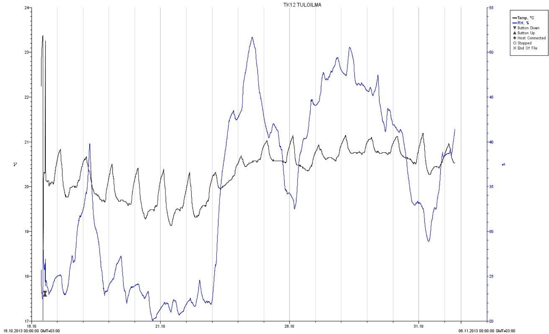
Kuva 10. IV-koneen TK2 tuloilman lämpötila- ja kosteustulokset 16.10-31.10 ajalta.
