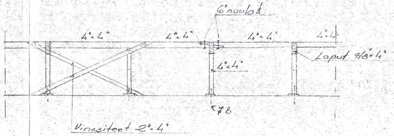
Yleiskuva orresta 1:50
