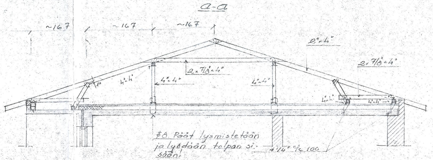
Yleiskuva orresta 1:50
